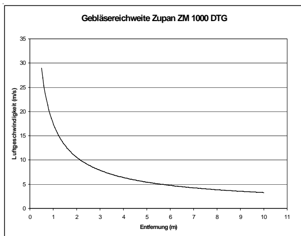
Abbildung 6: Gebläseerreichweite
