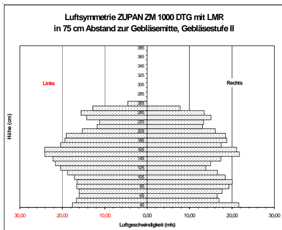
Abbildung 7: Luftgeschwindigkeiten in 75 cm Abstand zur Gebläsemitte
